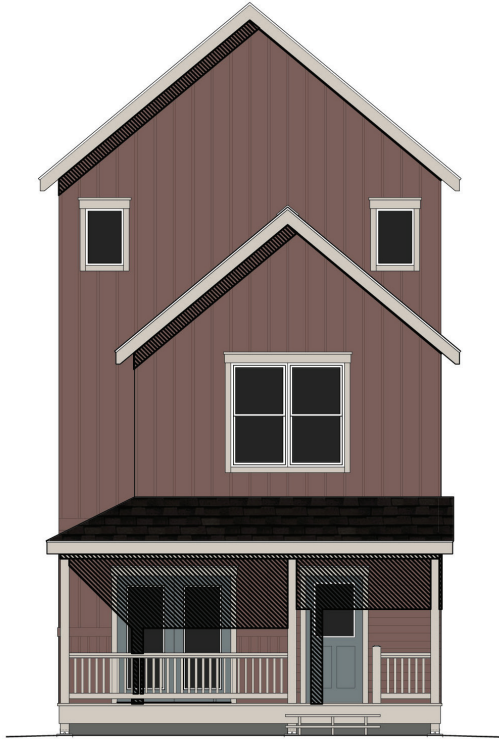
ELEVATION A
